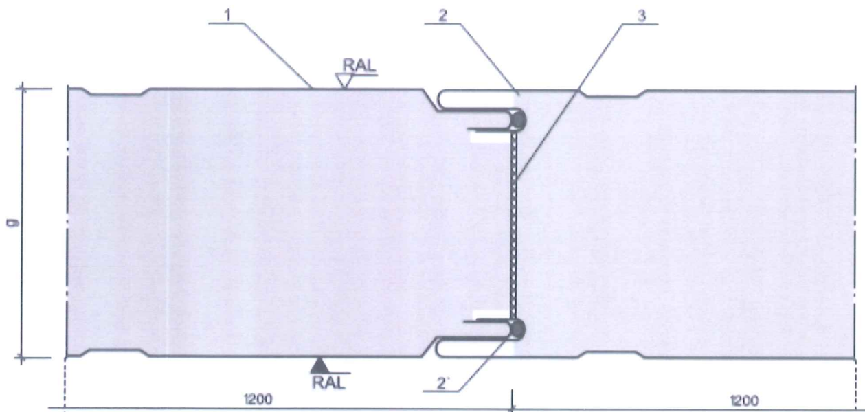
Rys.1 Płyta warstwowa BAAS-PANEL (rysunek dostarczony przez Zleceniodawcę)
